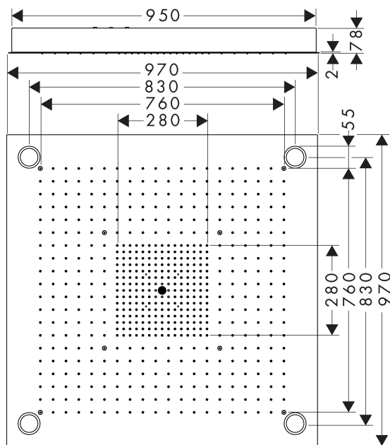
Kótovaný výkres
